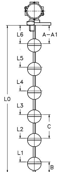
DN = UNI - DIN - ANSI flanges
